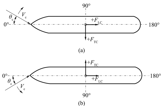
图 F.0.1 作用于船舶上的水动力示意图
